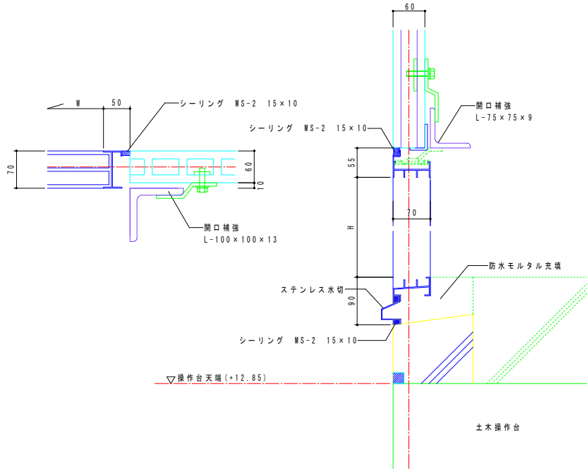
AD-1詳細図 1:5
