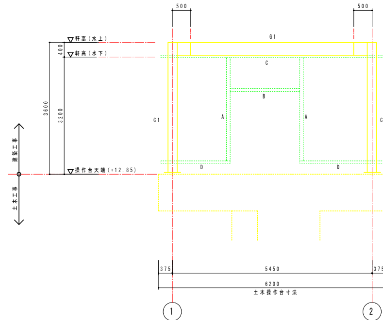
B通り軸組図 1 : 50
