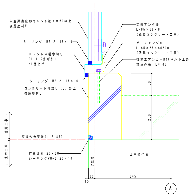
下部水切廻り詳細図 1:5
