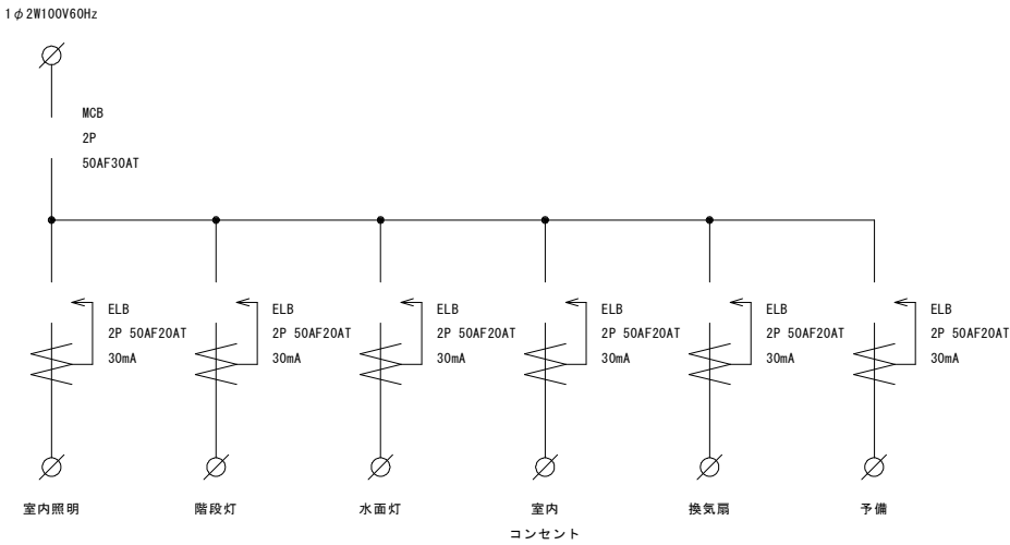
操作室棟 電灯分電盤 系統図
