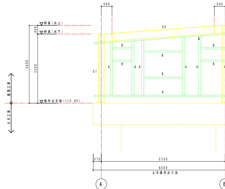
2通り軸組図 1 : 50
