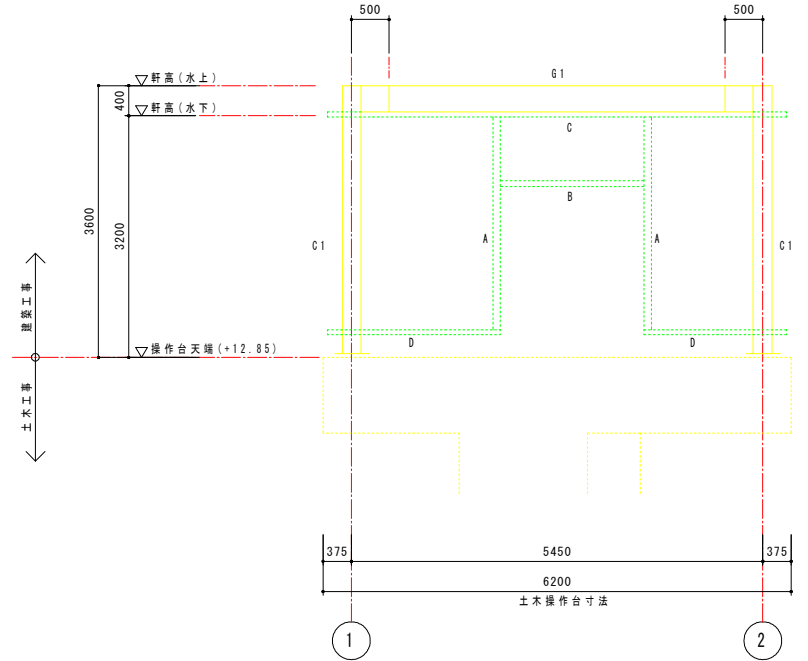
B通り軸組図 1:50
