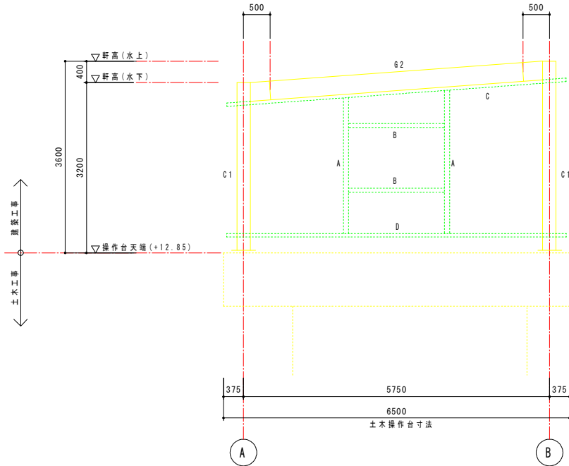
1,2通り軸組図 1:50
