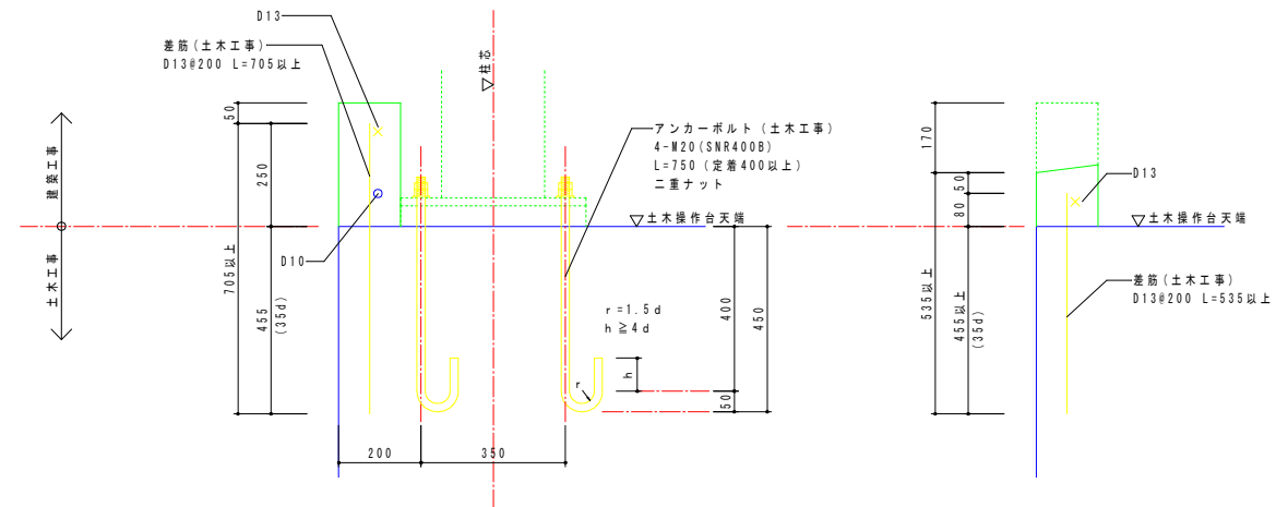
アンカーボルト・差筋詳細図 1:10
