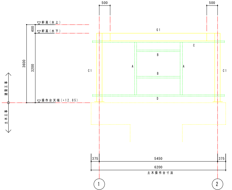
A通り軸組図 1:50
