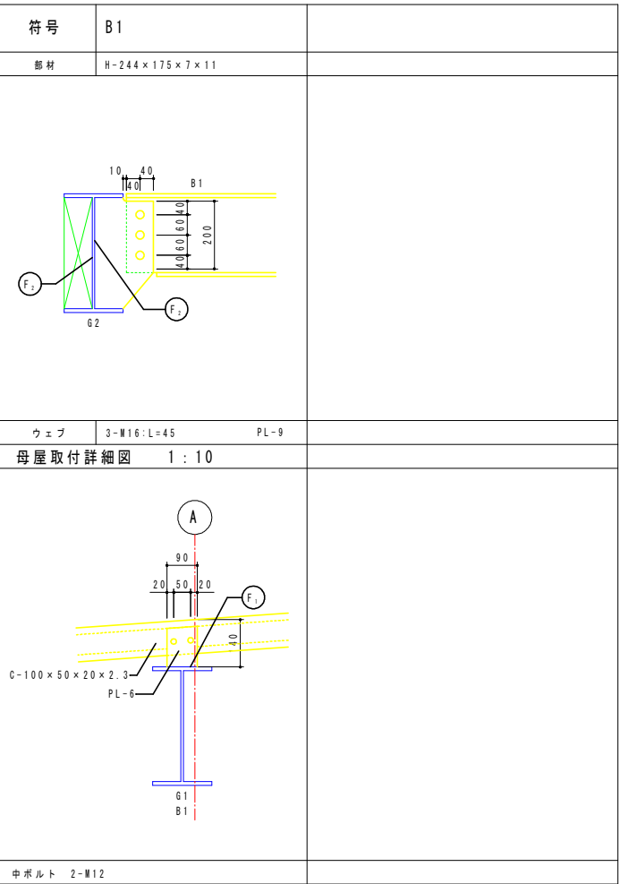
小梁継手リスト (ピン接合) 1:10 鋼種 SS400 高力ボルト F8T
