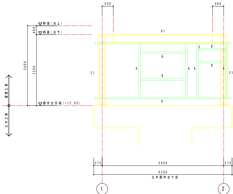
A通り軸組図 1 : 50
