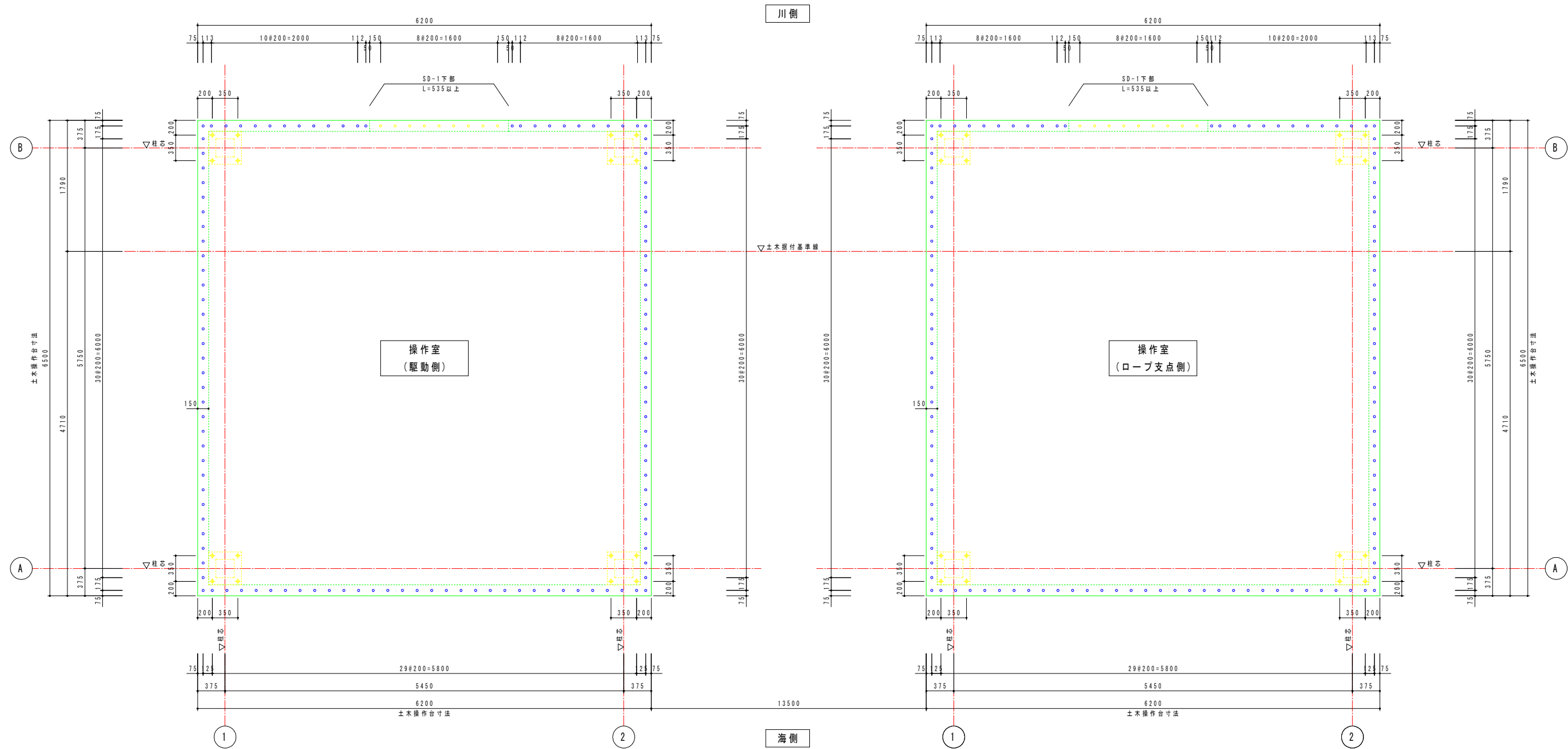
上屋差筋図 1:30
