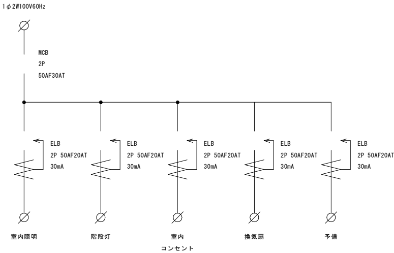
発電機棟 電灯分電盤 系統図
