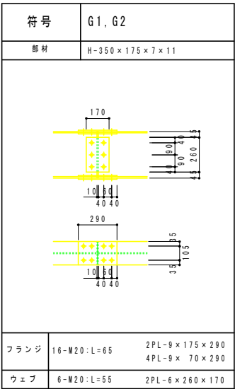
各部継手リスト S=1:10、20 鋼種 SS400 高力ボルト F8T
