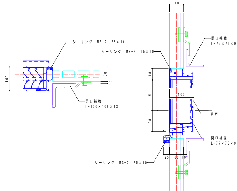
AG-1廻り詳細図 1:5
