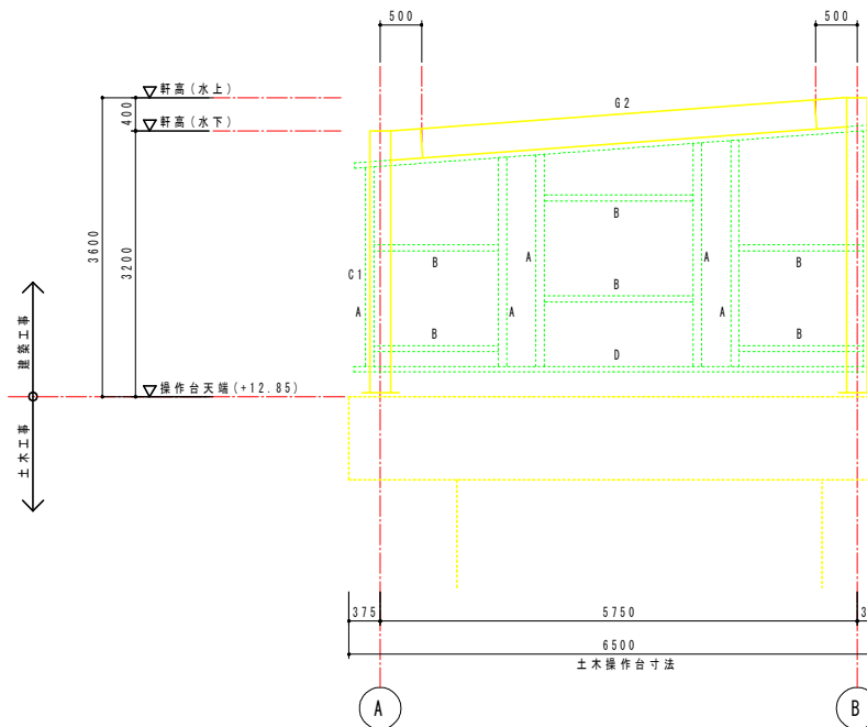
1通り軸組図 1 : 50
